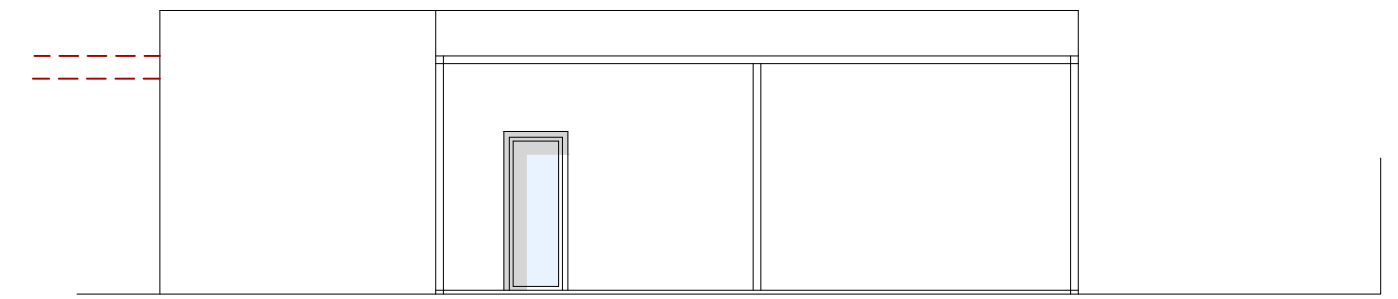
FAÇANA NORD 1/100
